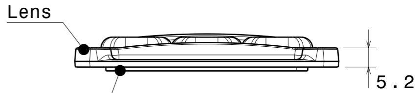
Front view Scale: 1:1
